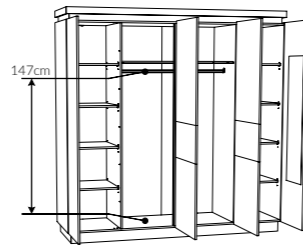
typ LYOV03L →/↑/↗ 59,7/198,1/42cm Square 2 Punkt – optionale Beleuchtung
