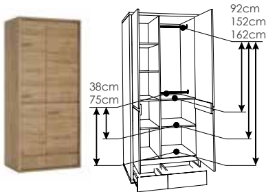
type 20 →/↑/↗ 86/197/58cm
