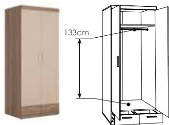
type 20 →/↑/↗ 80/195/60,8cm
